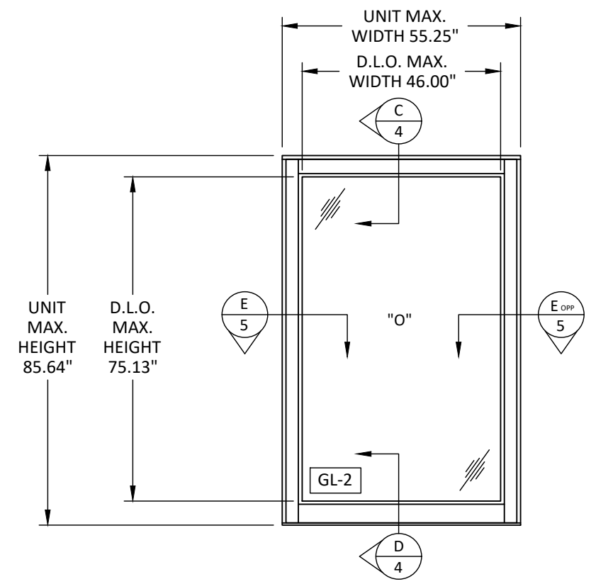
ELEVATION
